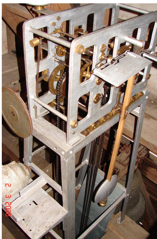
13. Mechanizm zegara wieżowego.
